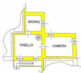
PIANO PRIMO
