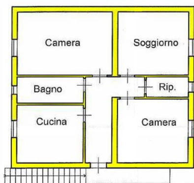
PIANO PRIMO
